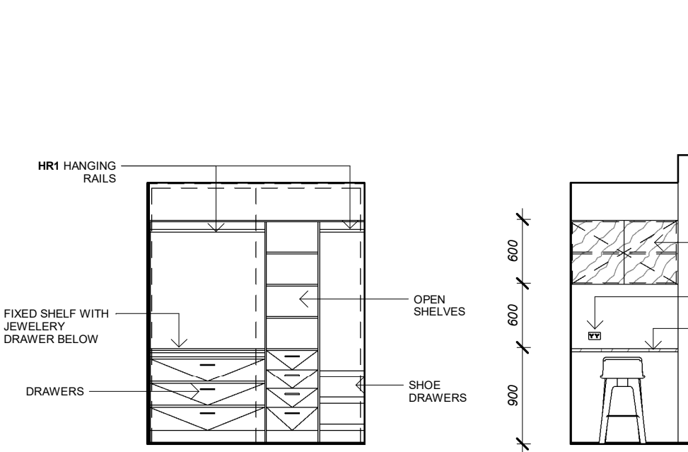
2.26 ELEVATION 1 : 50
