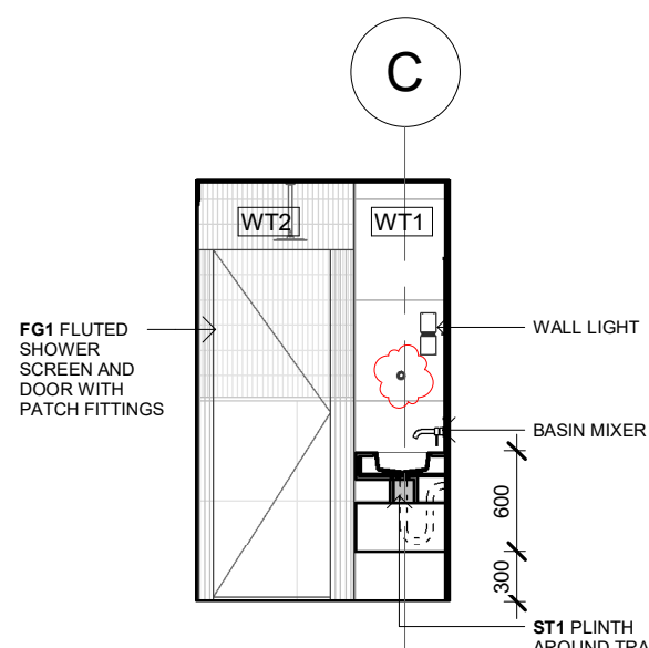
2.4 ELEVATION 1 : 50
