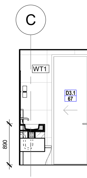
2.2 ELEVATION 1 : 50
