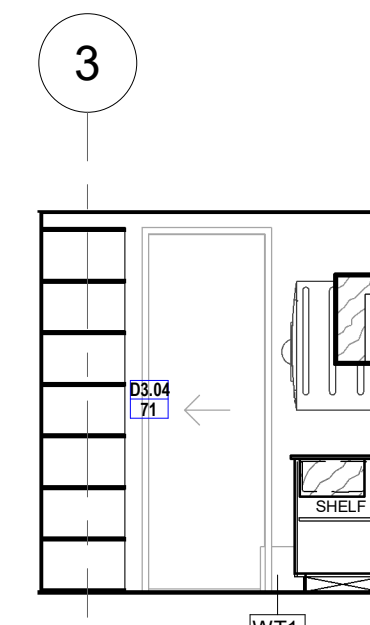
2.10 ELEVATION 1 : 50
