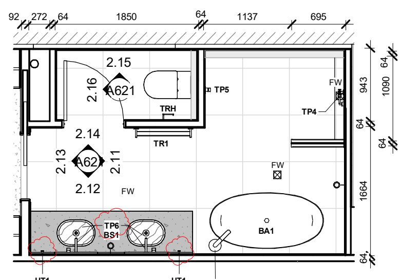
3 UNIT 2,4,6 ENSUITE 1 : 50 on A1 / 1 : 100 on A3
