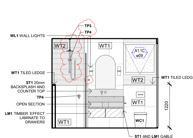
2.1 ELEVATION 1 : 50
