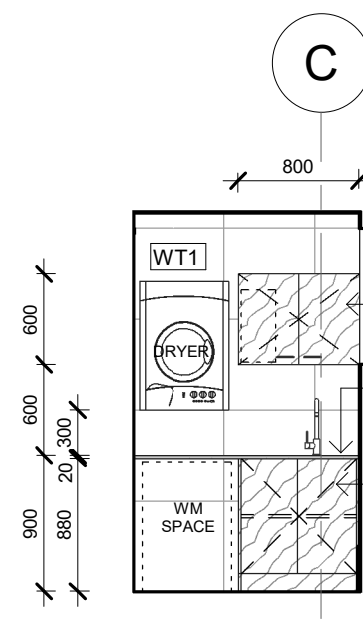
2.7 ELEVATION 1 : 50
