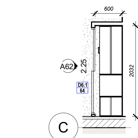
4 UNIT 2,4,6 ROBE 2 1 : 50 on A1 / 1 : 100 on A3
