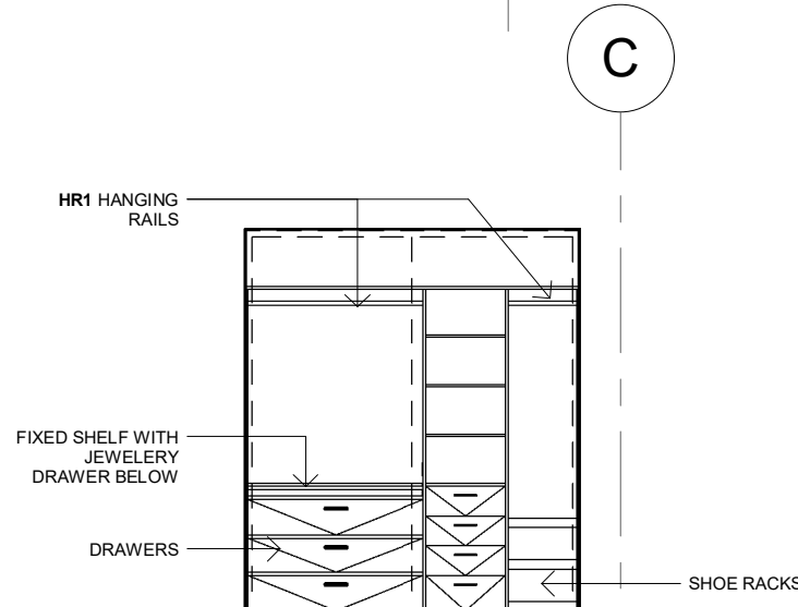
2.25 ELEVATION 1 : 50
