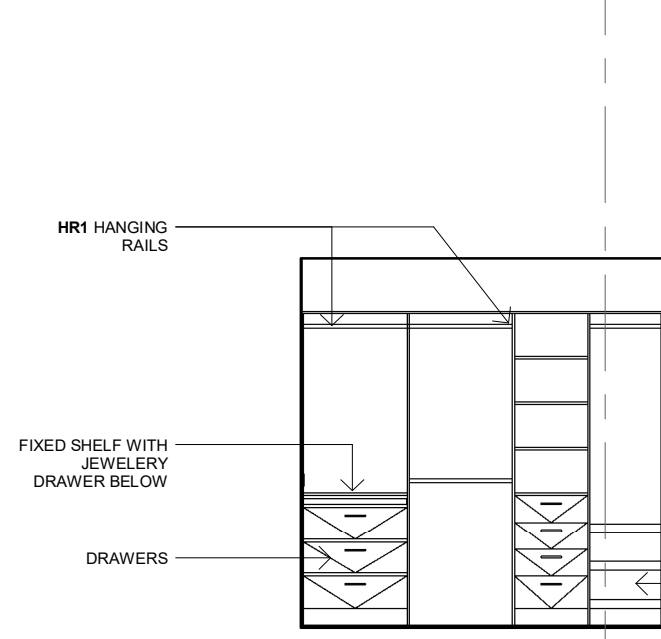
2.23 ELEVATION 1 : 50
