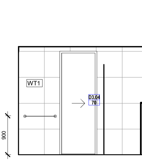
2.3 ELEVATION 1 : 50
