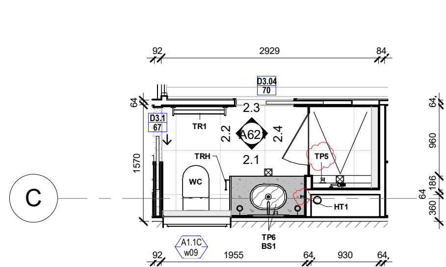
1 UNIT 2,4,6 BATHROOM 1 : 50 on A1 / 1 : 100 on A3
