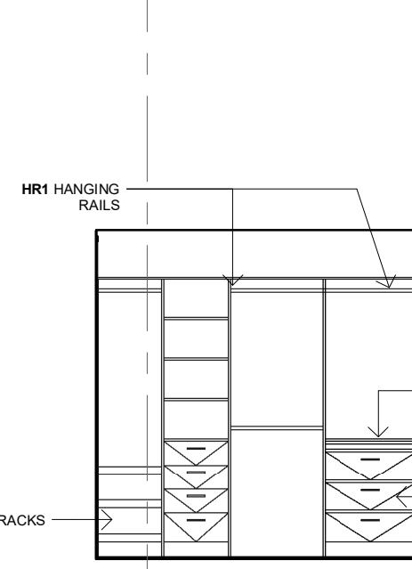
2.24 ELEVATION 1 : 50
