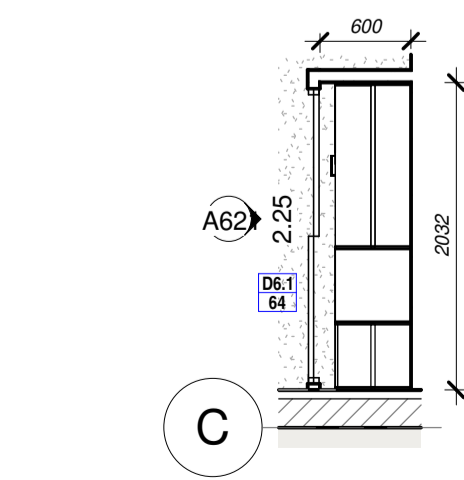
4 UNIT 2,4,6 ROBE 2 1 : 50 on A1 / 1 : 100 on A3
