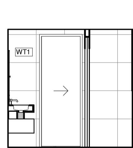
2.13 ELEVATION 1 : 50
