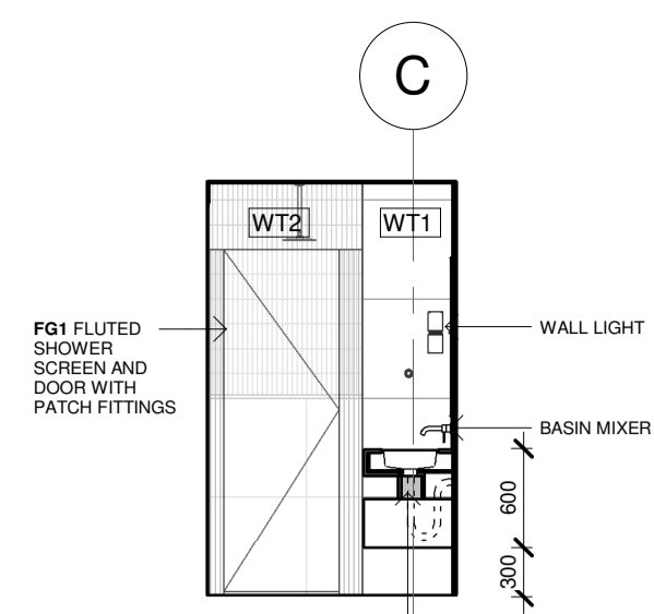
2.4 ELEVATION 1 : 50
