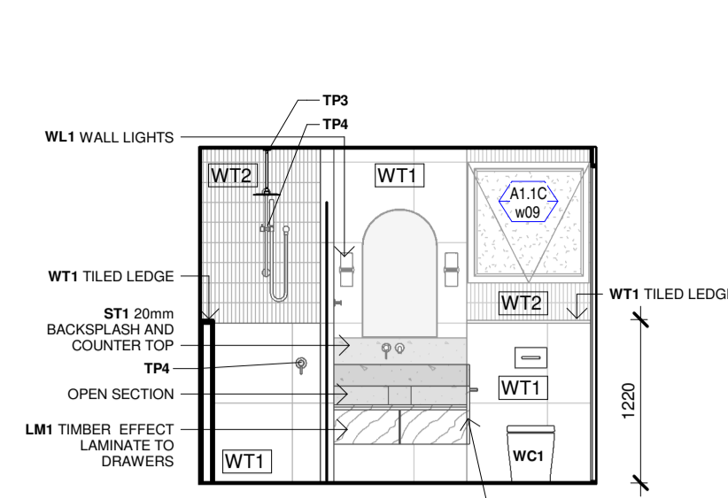
2.1 ELEVATION 1 : 50
