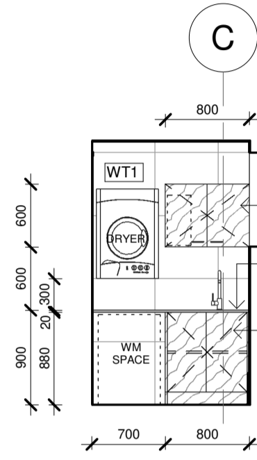
2.7 ELEVATION 1 : 50
