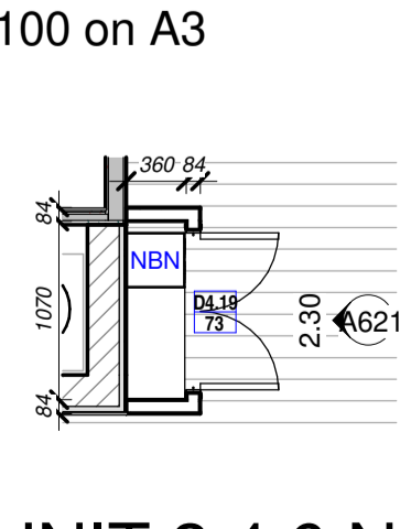
7 UNIT 2,4,6 NBN 1 : 50 on A1 / 1 : 100 on A3
