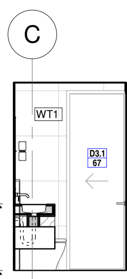
2.2 ELEVATION 1 : 50
