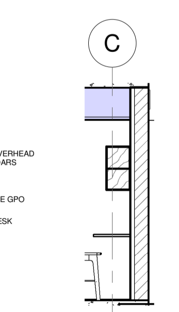
2.28 SECTION 1 : 50
