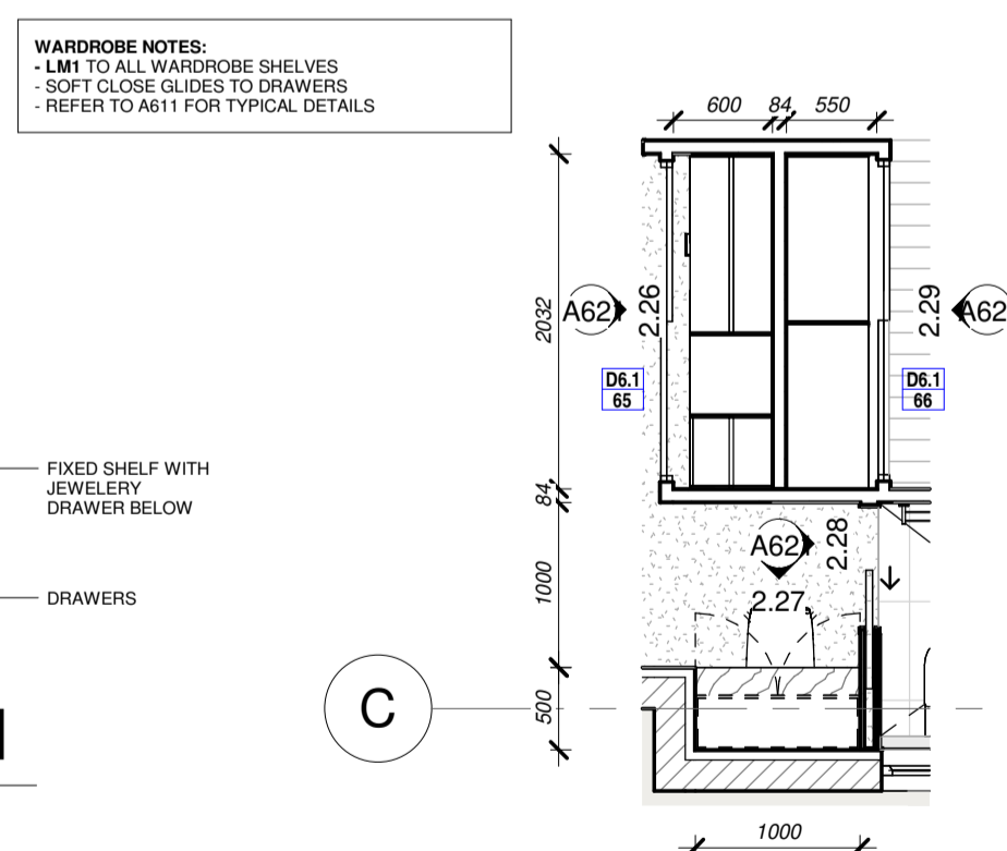
6 UNIT 2,4,6 ROBE 3+STUDY+STORE 1 : 50 on A1 / 1 : 100 on A3
