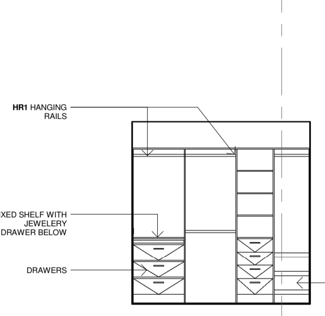
2.23 ELEVATION 1 : 50
