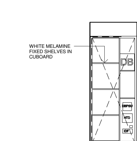
2.30 ELEVATION 1 : 50
