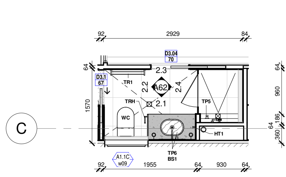
1 UNIT 2,4,6 BATHROOM 1 : 50 on A1 / 1 : 100 on A3
