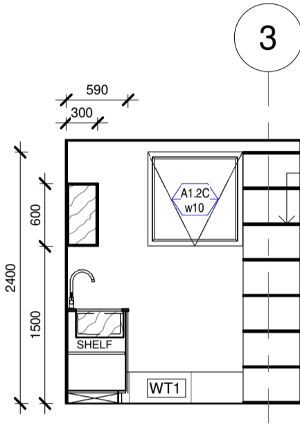
2.8 ELEVATION 1 : 50
