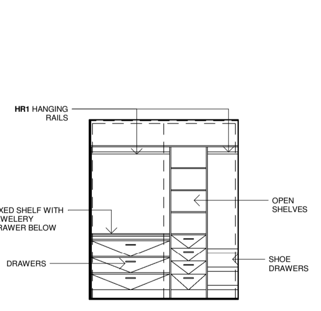
2.26 ELEVATION 1 : 50
