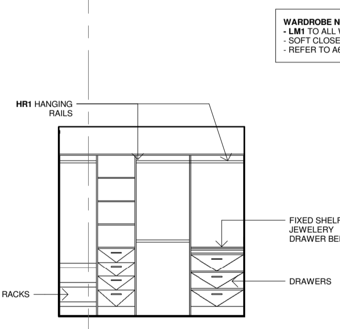
2.24 ELEVATION 1 : 50
