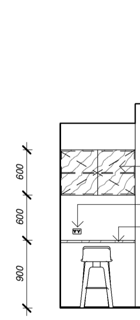
2.27 ELEVATION 1 : 50
