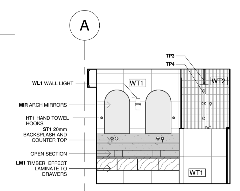
3.15 ELEVATION 1 : 50
