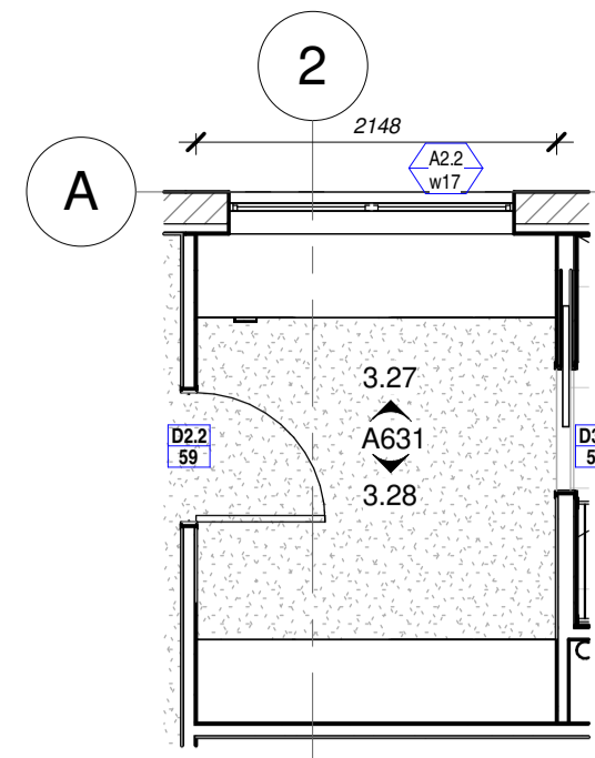
2 UNIT 3,5,7 ROBE 1 1 : 50 on A1 / 1 : 100 on A3
