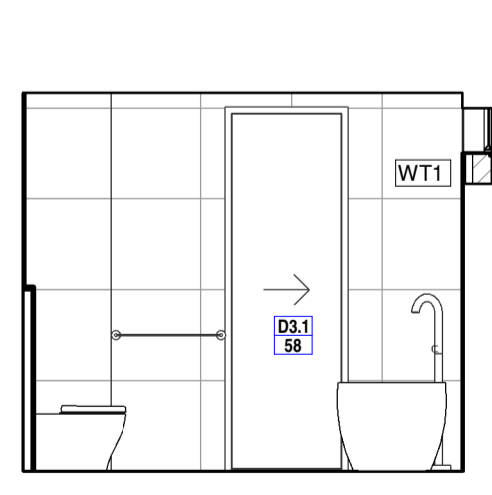
3.17 ELEVATION 1 : 50
