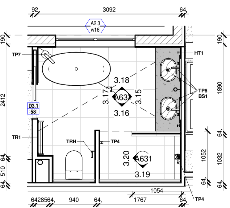
3 UNIT 3,5,7 ENSUITE 1 : 50 on A1 / 1 : 100 on A3
