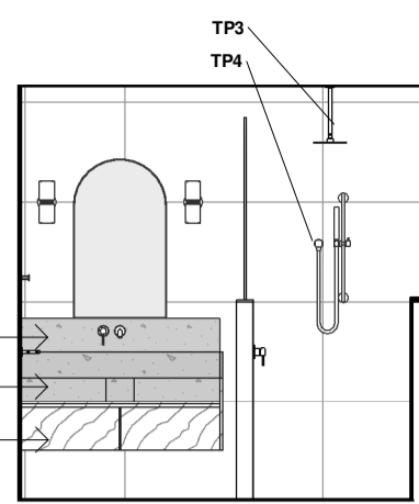
3.2 ELEVATION 1 : 50
