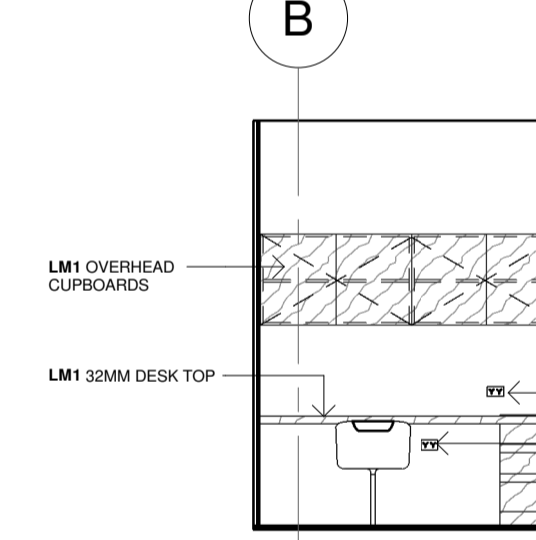
3.13 ELEVATION 1 : 50
