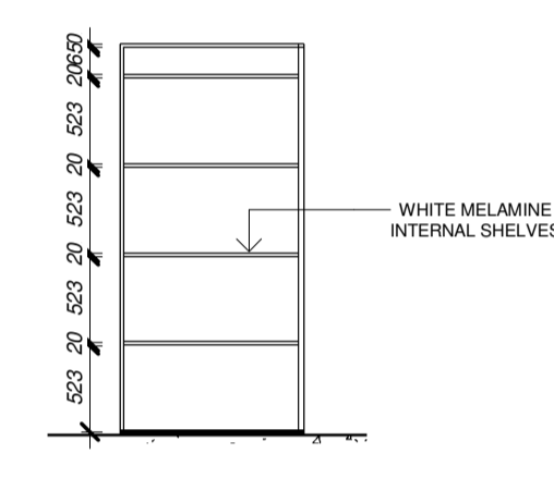
3.36 ELEVATION 1 : 50
