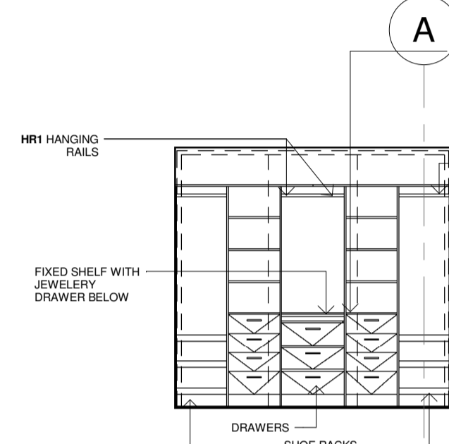
3.30 ELEVATION 1 : 50
