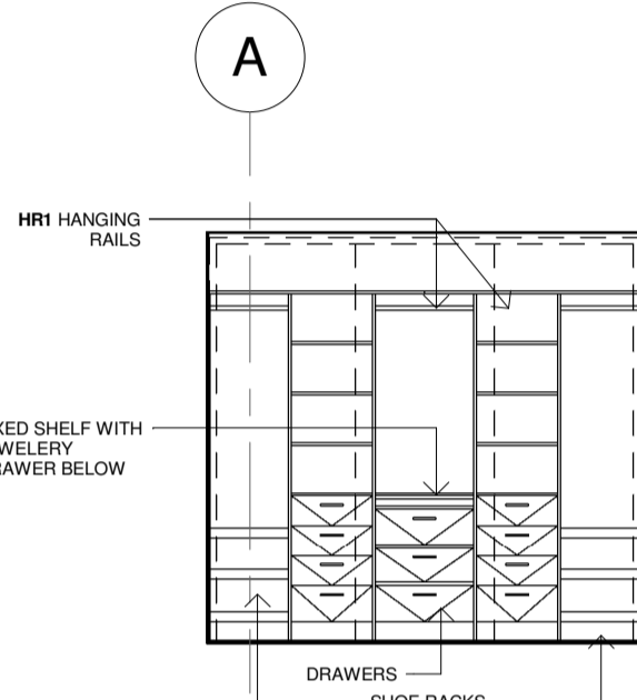
3.29 ELEVATION 1 : 50
