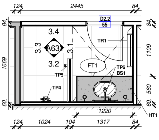
1 UNIT 3,5,7 BATHROOM 1 : 50 on A1 / 1 : 100 on A3
