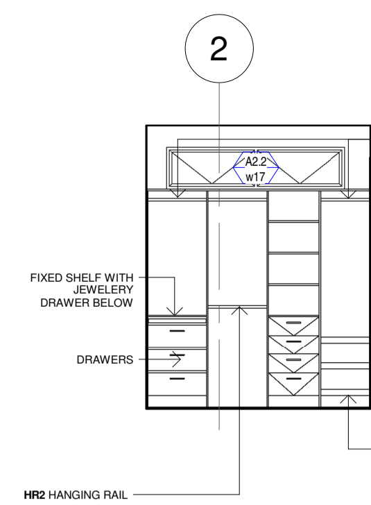
3.27 ELEVATION 1 : 50
