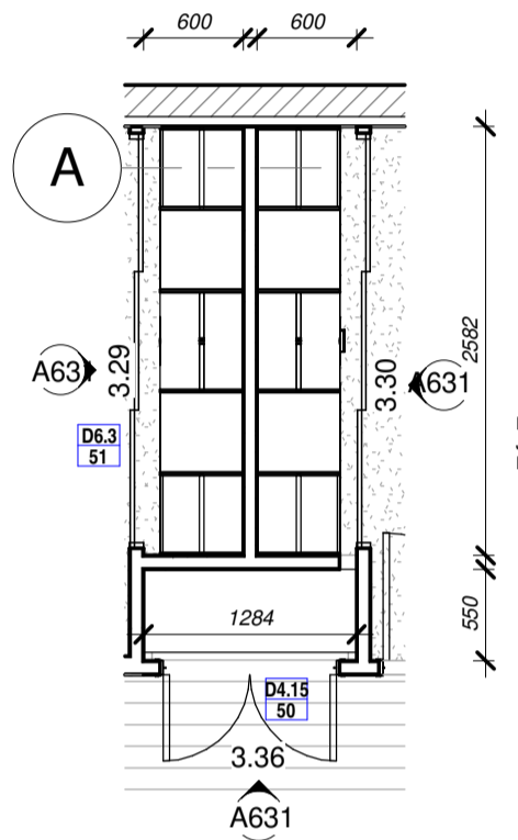
4 UNIT 3,5,7 ROBE 2 1 : 50 on A1 / 1 : 100 on A3
