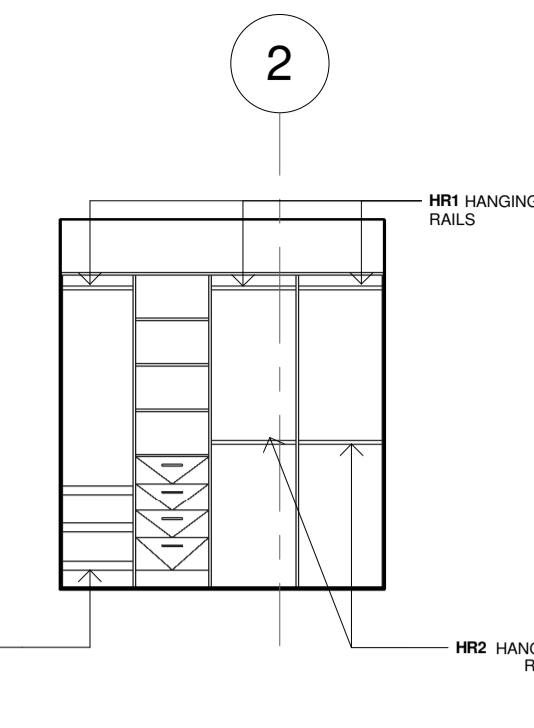
3.28 ELEVATION 1 : 50
