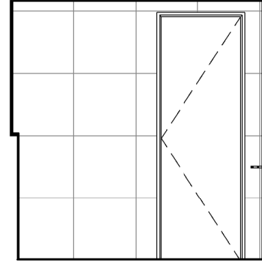
3.4 ELEVATION 1 : 50
