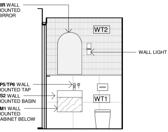
3.32 ELEVATION 1 : 50
