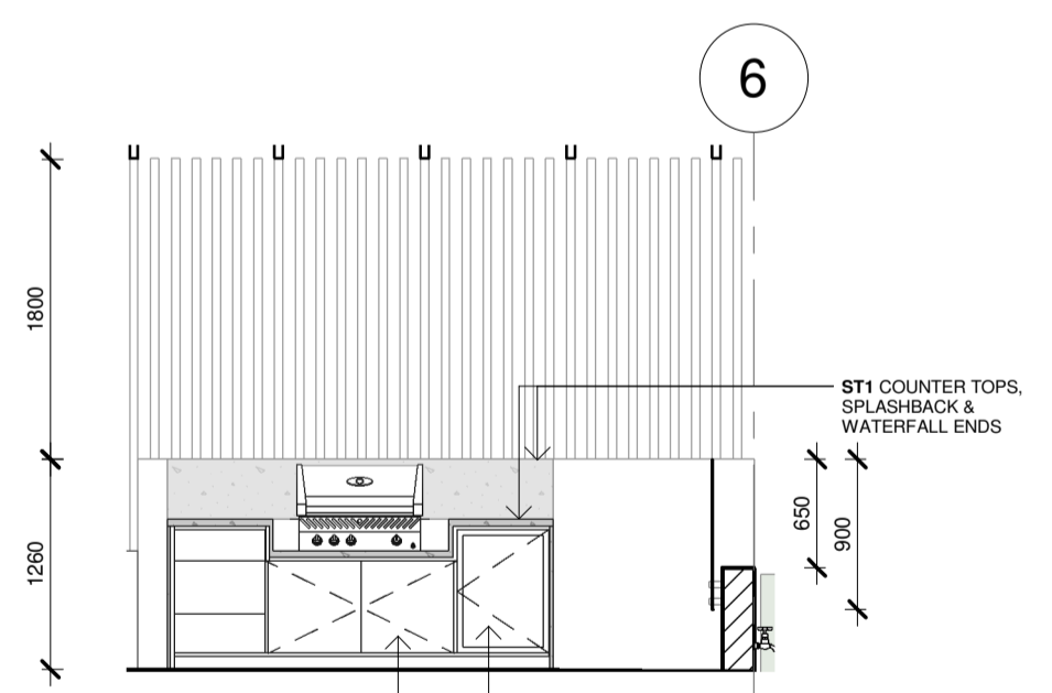
1.9 ELEVATION 1 : 50
