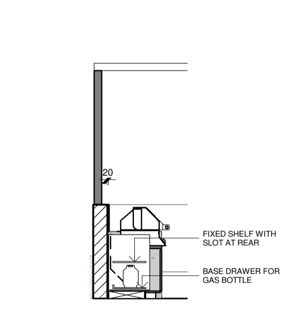
1.10 ELEVATION 1 : 50
