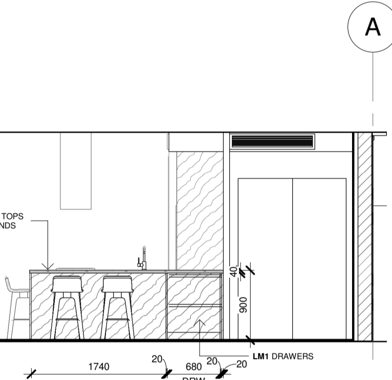
8.32 ELEVATION 1 : 50
