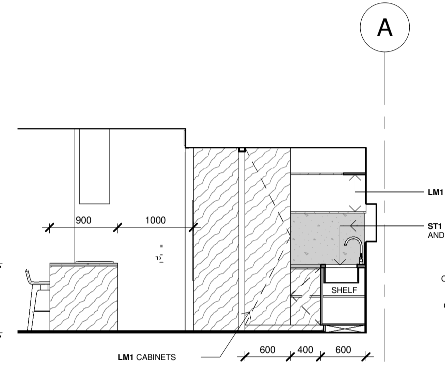
8.30 ELEVATION 1 : 50
