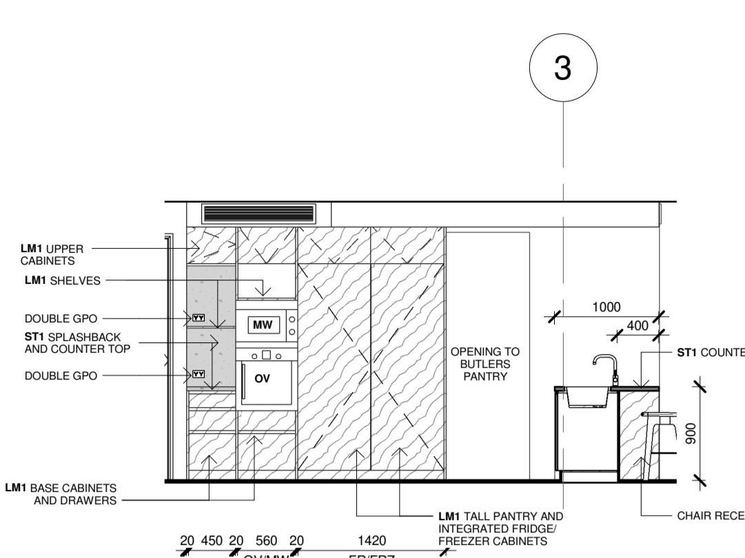
8.25 ELEVATION 1 : 50
