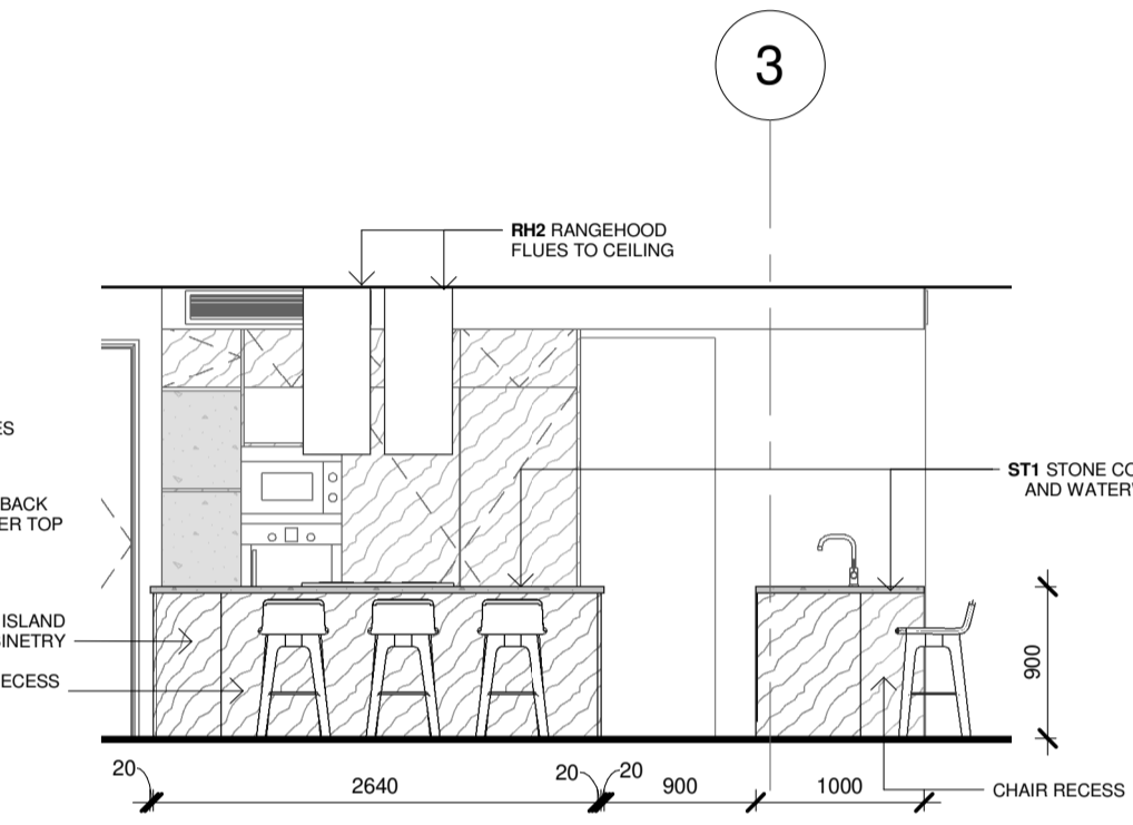
8.31 ELEVATION 1 : 50
