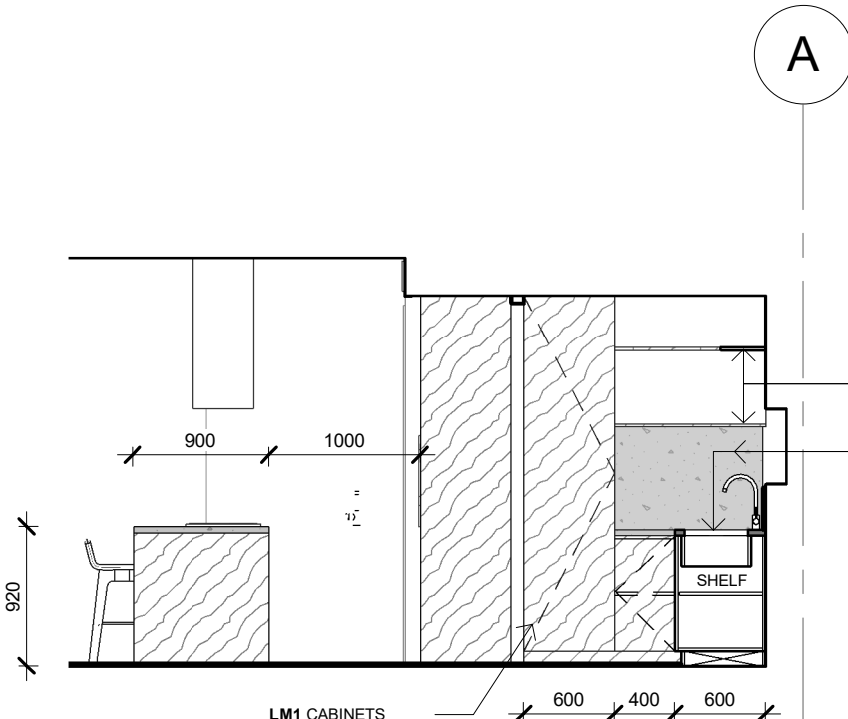
8.30 ELEVATION 1 : 50
