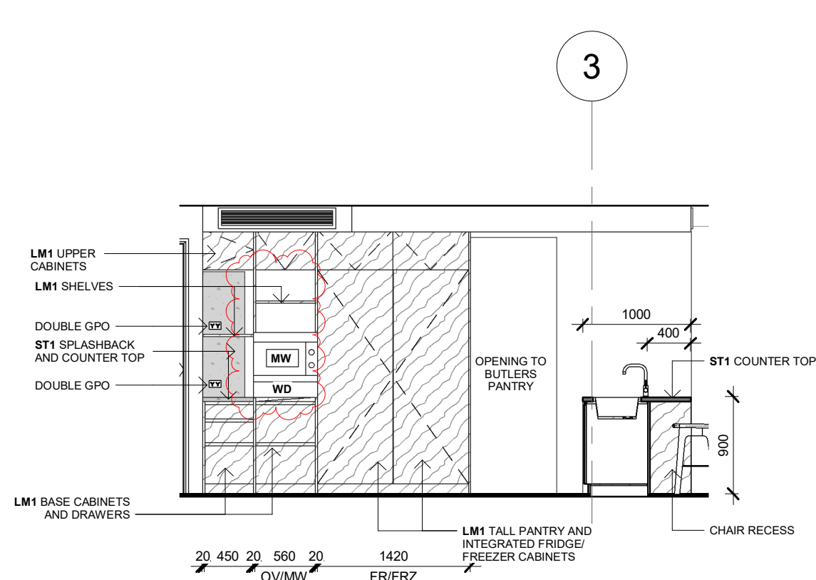
8.25 ELEVATION 1 : 50
