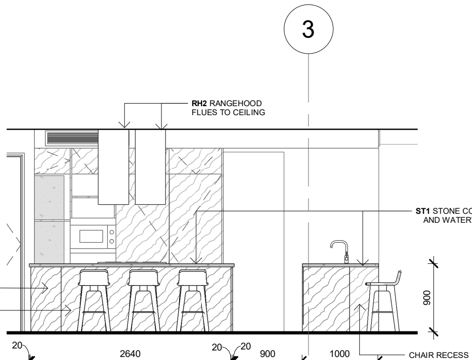
8.31 ELEVATION 1 : 50
