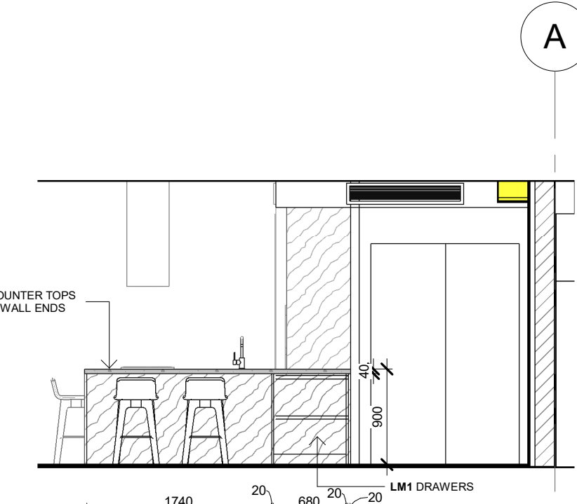
8.32 ELEVATION 1 : 50
