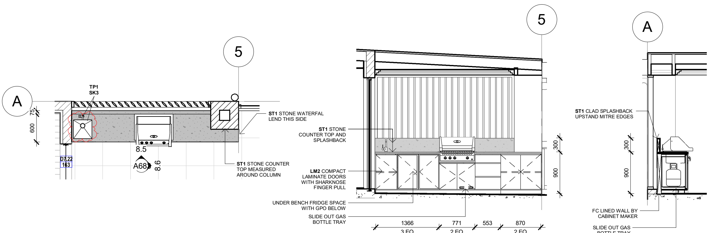
2 UNIT 8 BBQ 1 : 50 on A1 / 1 : 100 on A3
